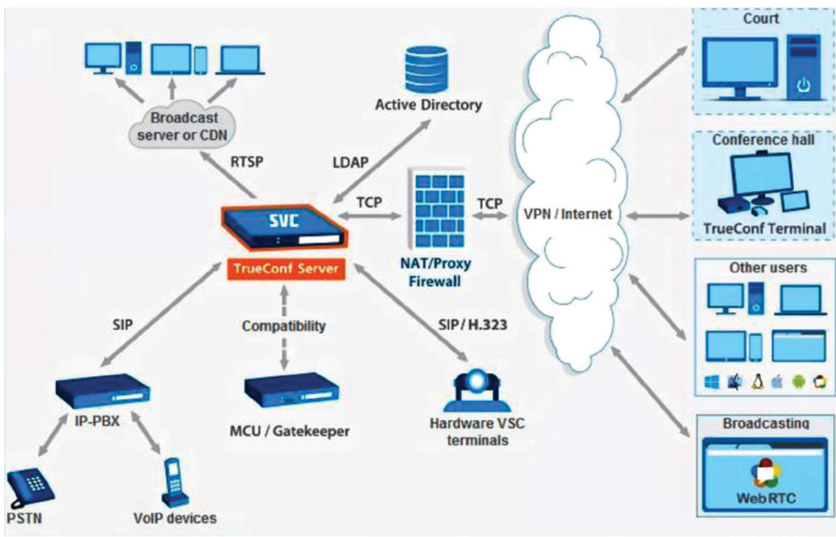
Figura 3. Schema de funcționare a serverului de videoconferință a sistemului TrueConf 64
